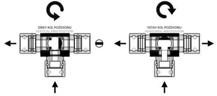
T TİPİ ÇALIŞMA PRENSİBİ T BORE WORKING PRINCIPLE
