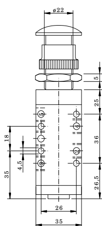
5/2 way
