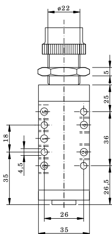
5/2 way
