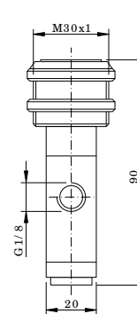
3/2 way
