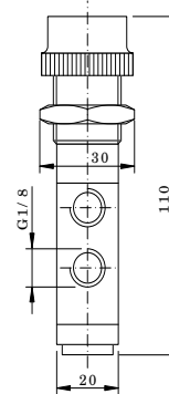
3/2 way
