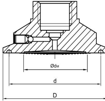
Kelepçe Bağlantılı PN 40 bar
